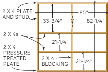
LEFT WALL
